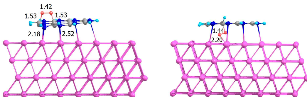
図1 理論計算によって求めた BN - 金表面に吸着した酸素の安定化構造
