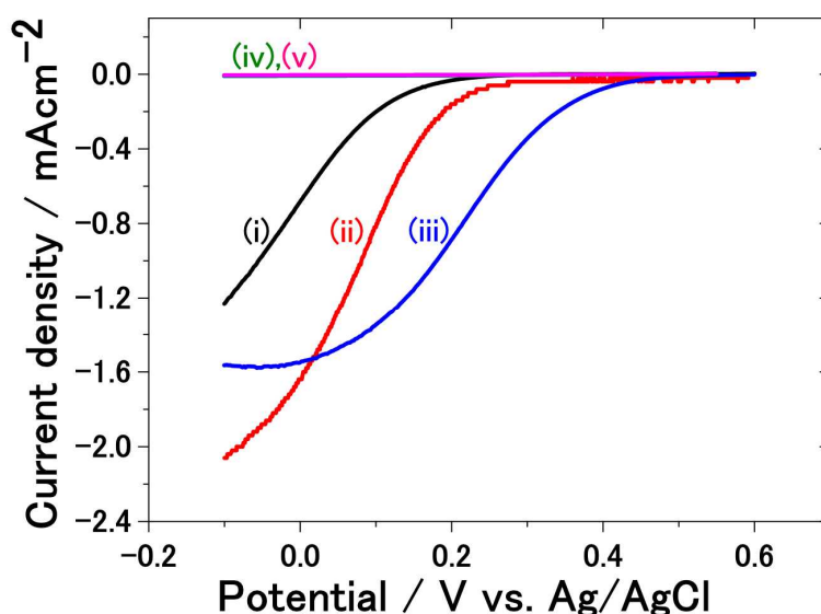
図3 回転電極法によって観測された酸素の還元反応にともなう電流応答曲線
