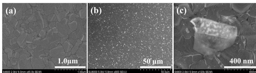
図2 金基板上に担持したBNナノシートの電子顕微鏡写真
